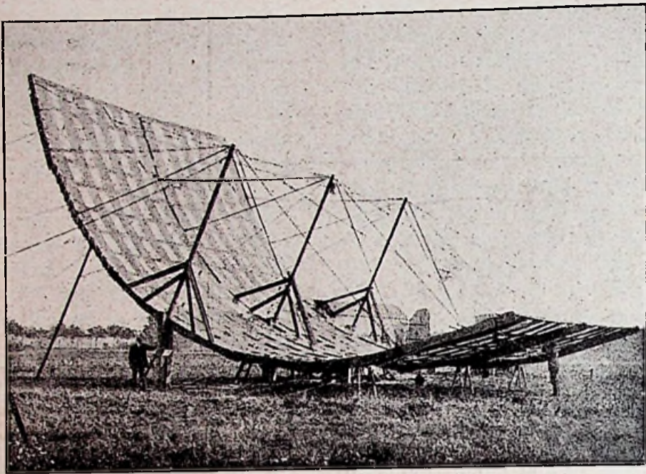
De reflector voor omhoog gerichte korte golven.
