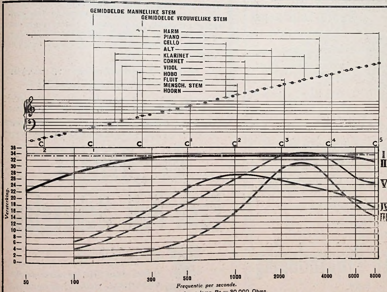
KARAKTERISTIEKEN VAN VERSCHILLENDE TRANSFORMATOREN. Kromme I = Volmaakt. Kromme II = Ferranti A F 3 Patent hoogfrequent transformator. Krommen III, IV en V = WELBEKENDE transformatoren van ANDERE FABRIKATEN.
